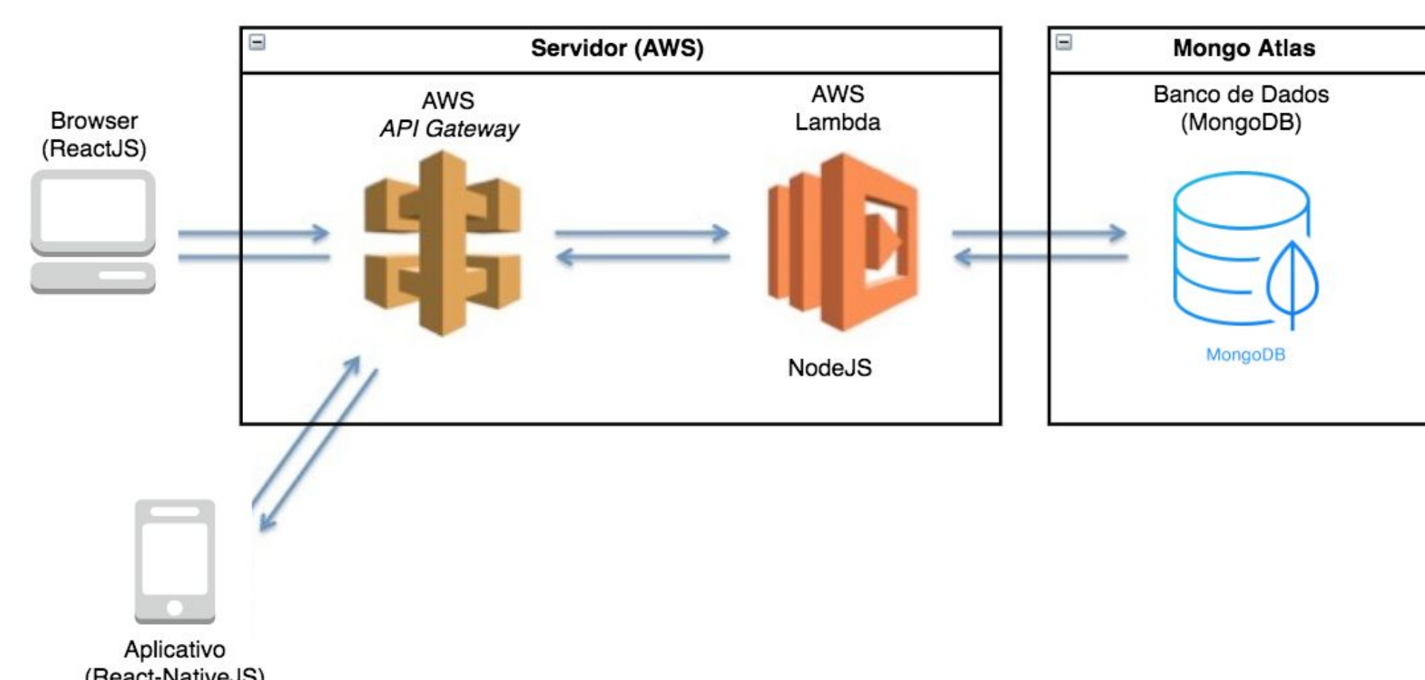
Figura 2 - Arquitetura do sistema.
